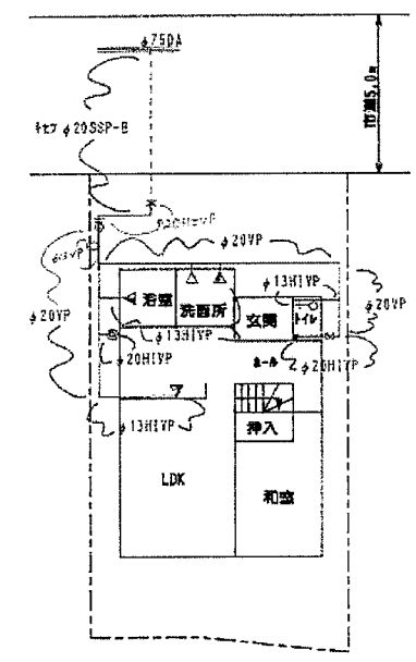
1階給水平面図
